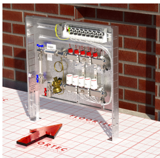
Einbau des Fertigverteilerschranks an gewünschte Wandposition
