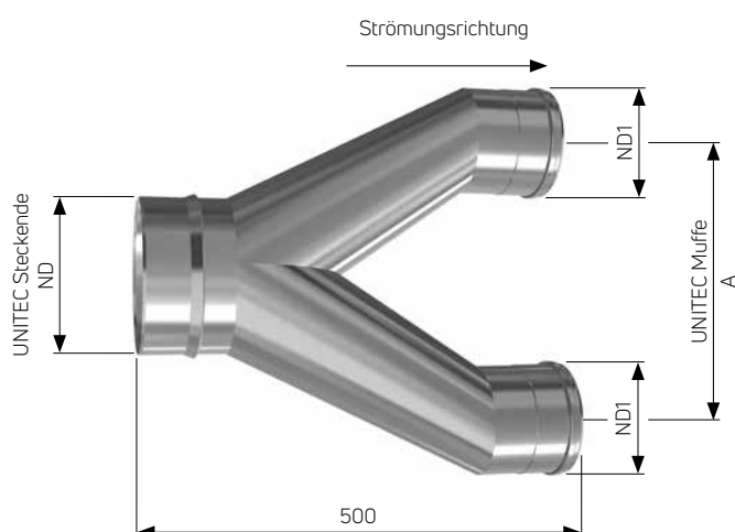
Maßtabelle
