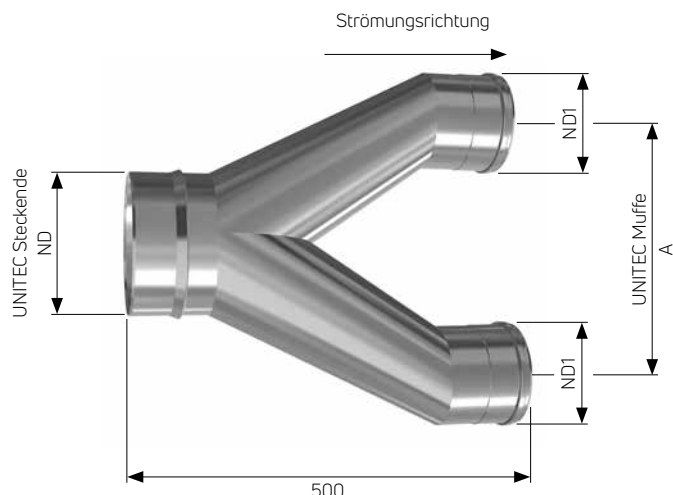
Maßtabelle
